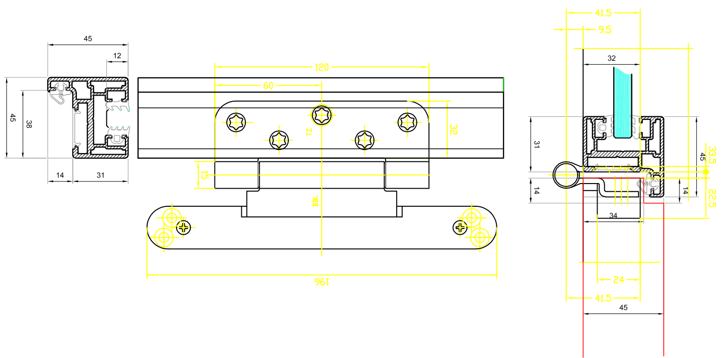
SIMONSWERK VN 2927/120 Compact Planum
