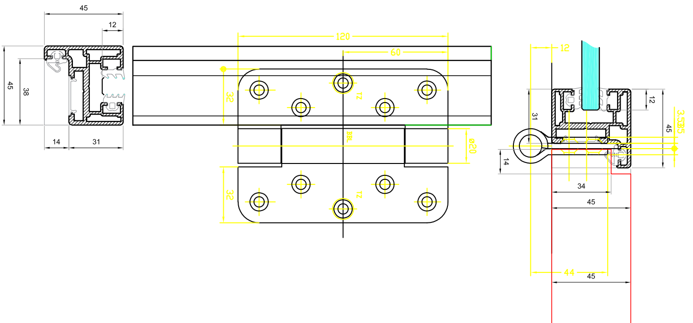
SIMONSWERK VN 2929/120
